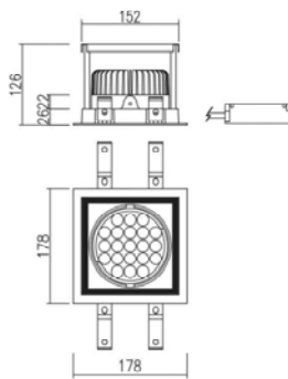
Technische Zeichnung
